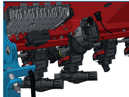
Düngerdosiersystem FertiSmart Mit ISM-Motor (Integrated Smart Motor) Ein Motor für mehrere Dosierer
