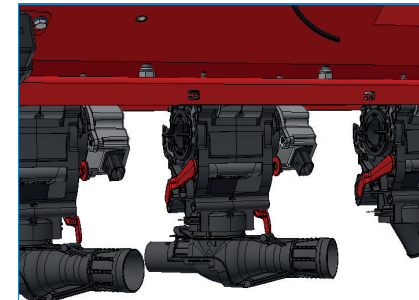
Düngerdosiersystem FertiSmart Mit MSM-Motor (Monosem Smart Motor) Ein Motor pro Dosierer
